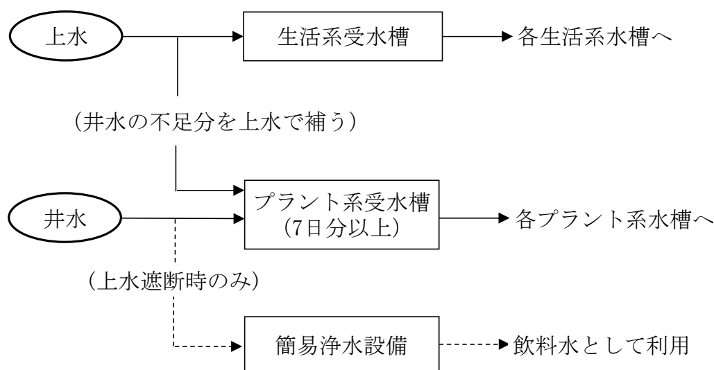
図 2.1 給水フロー（参考）
